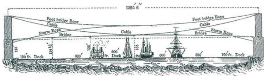
Alzado del puente mostrando las cuerdas temporales utilizadas para el sistema de cables.
