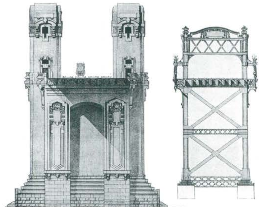
Detalle de la pila. Dibujo tomado de [194]
