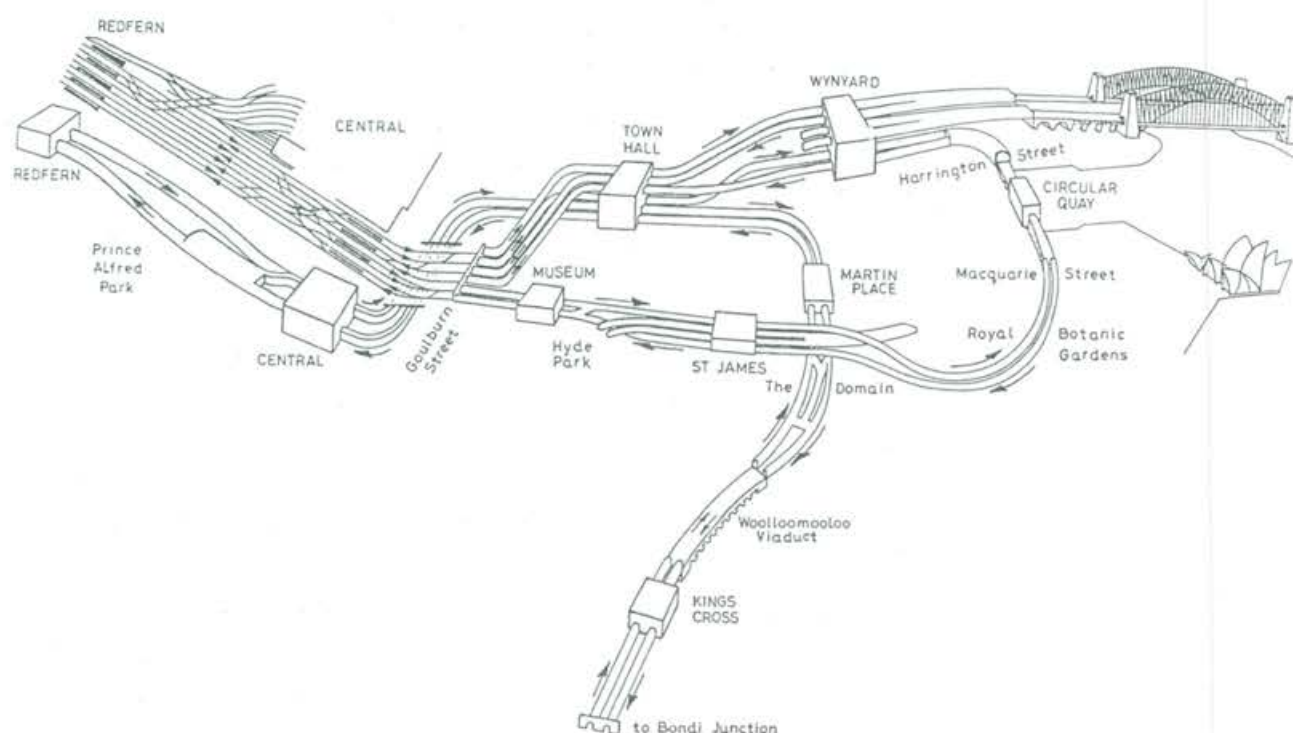
Red de túneles de metro [23:91]
