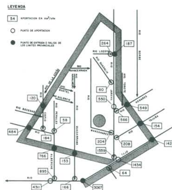
Aportaciones en régimen natural
