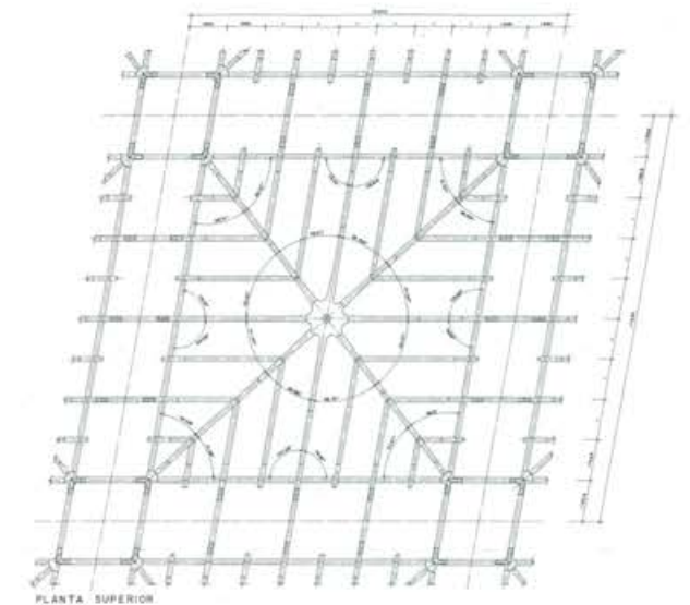
PLANTA SUPERIOR
