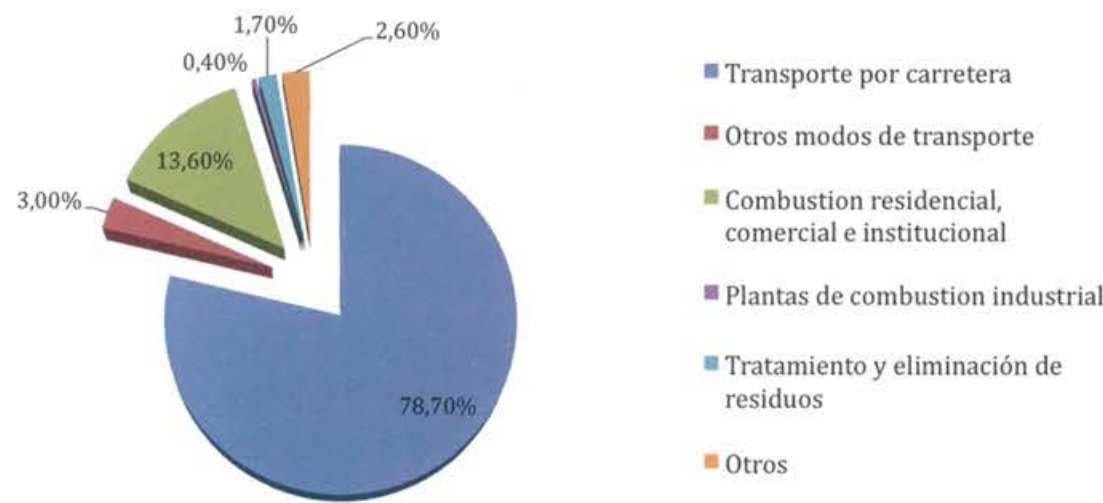
Distribución de emisiones de PM10 por sectores
