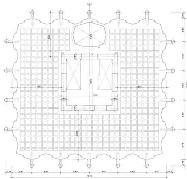
planta tipo
