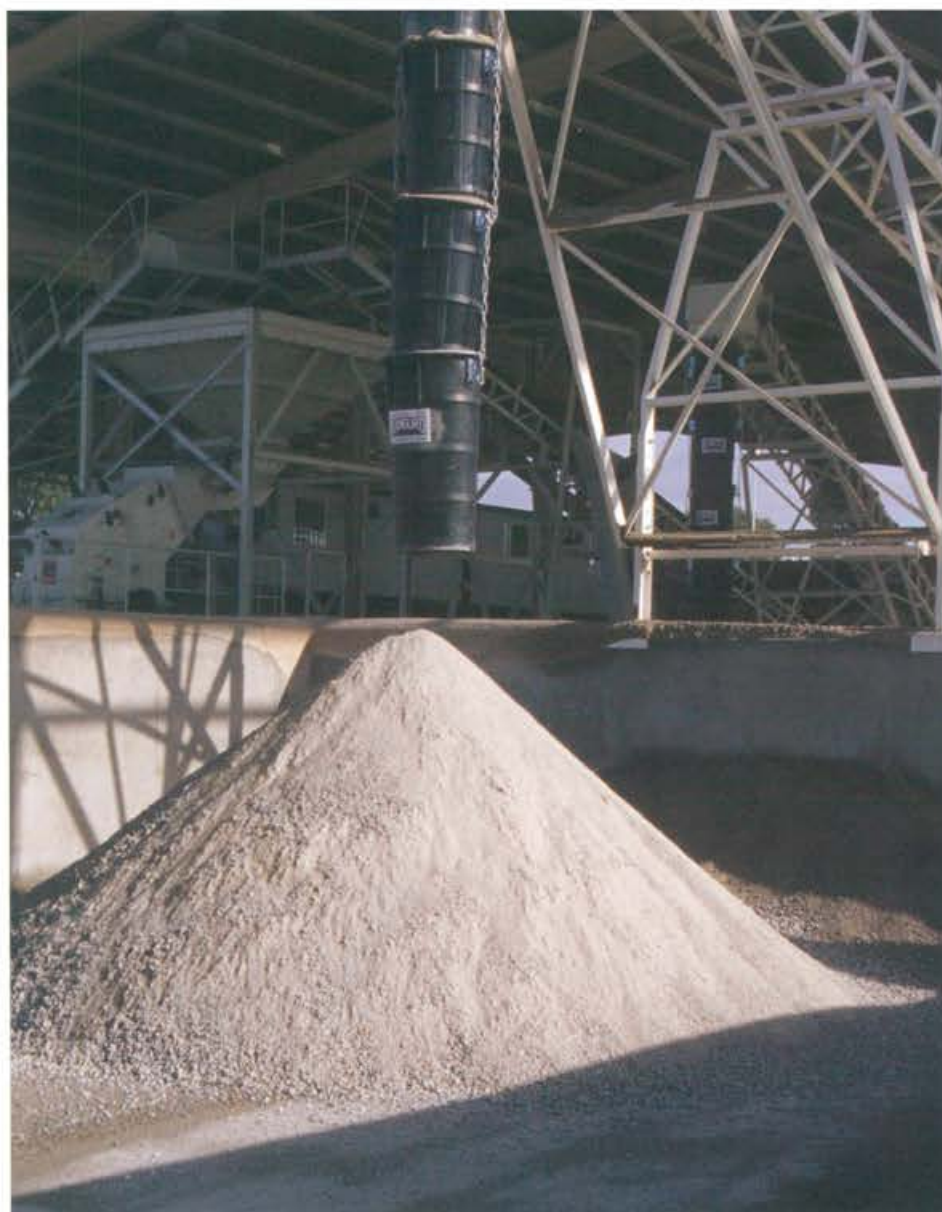
Árido reciclado en la planta de residuos de construcción y demolición de Navacarnero
