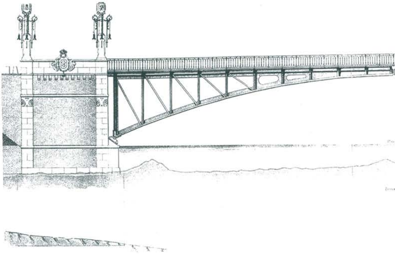
Puente de la Princesa de Asturias en Madrid (Machimbarrena y Beamonte, 1910) [146:1]
