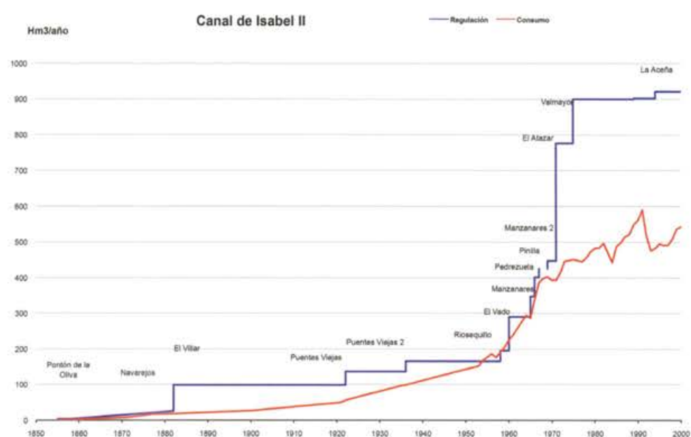
Evolución de demanda y capacidad del Canal
