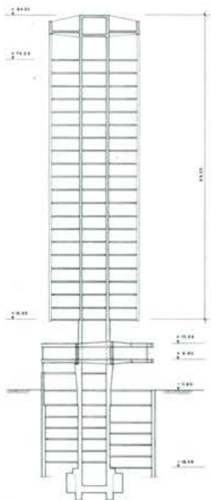
alzado sección
