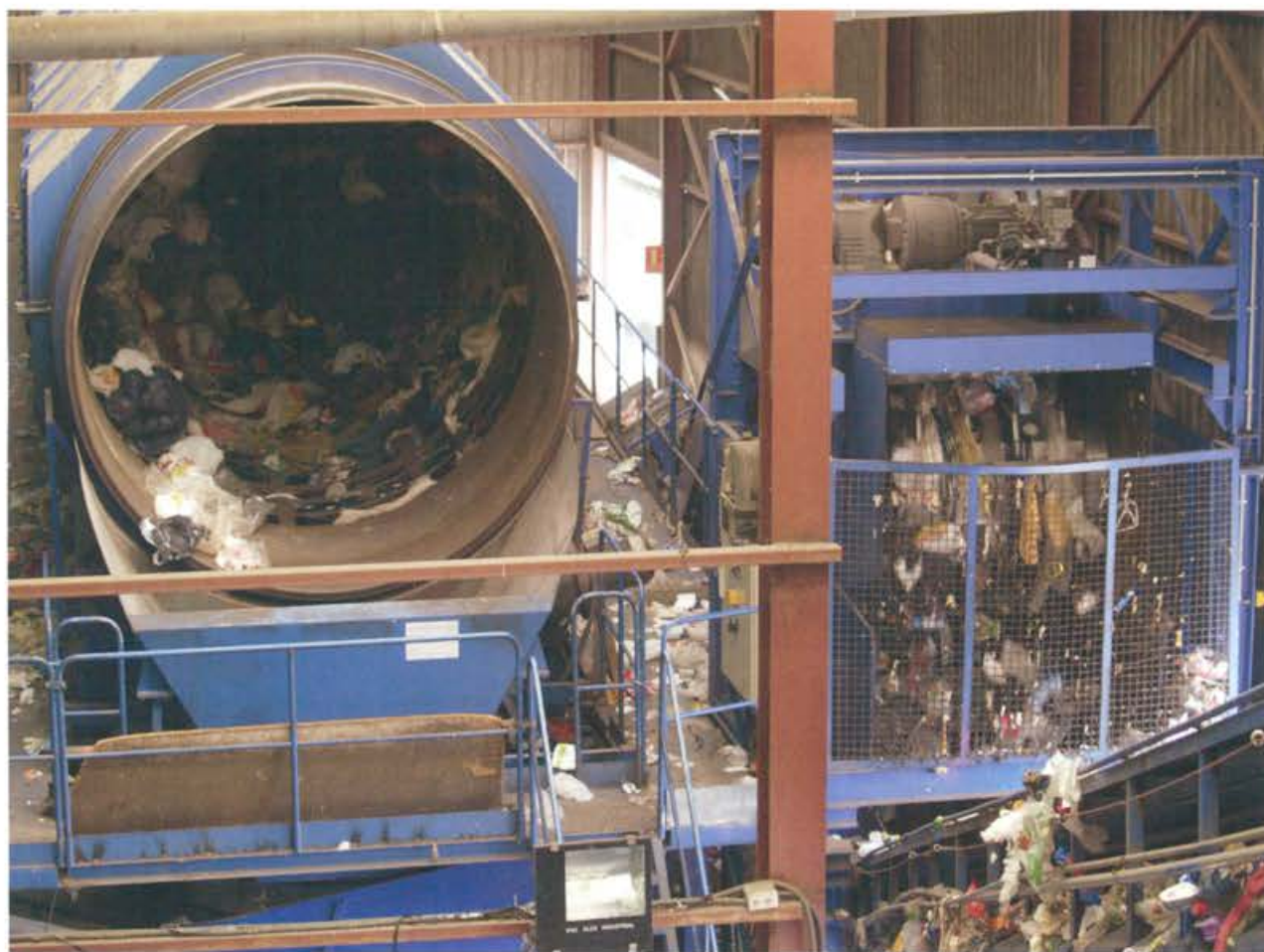
Trómel de separación volumétrica de la Planta de Clasificación de Envases de Pinto
