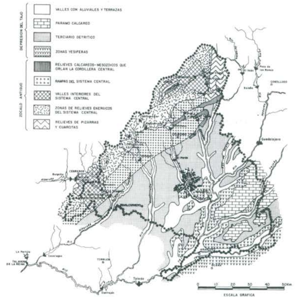
Geomorfología de Madrid
