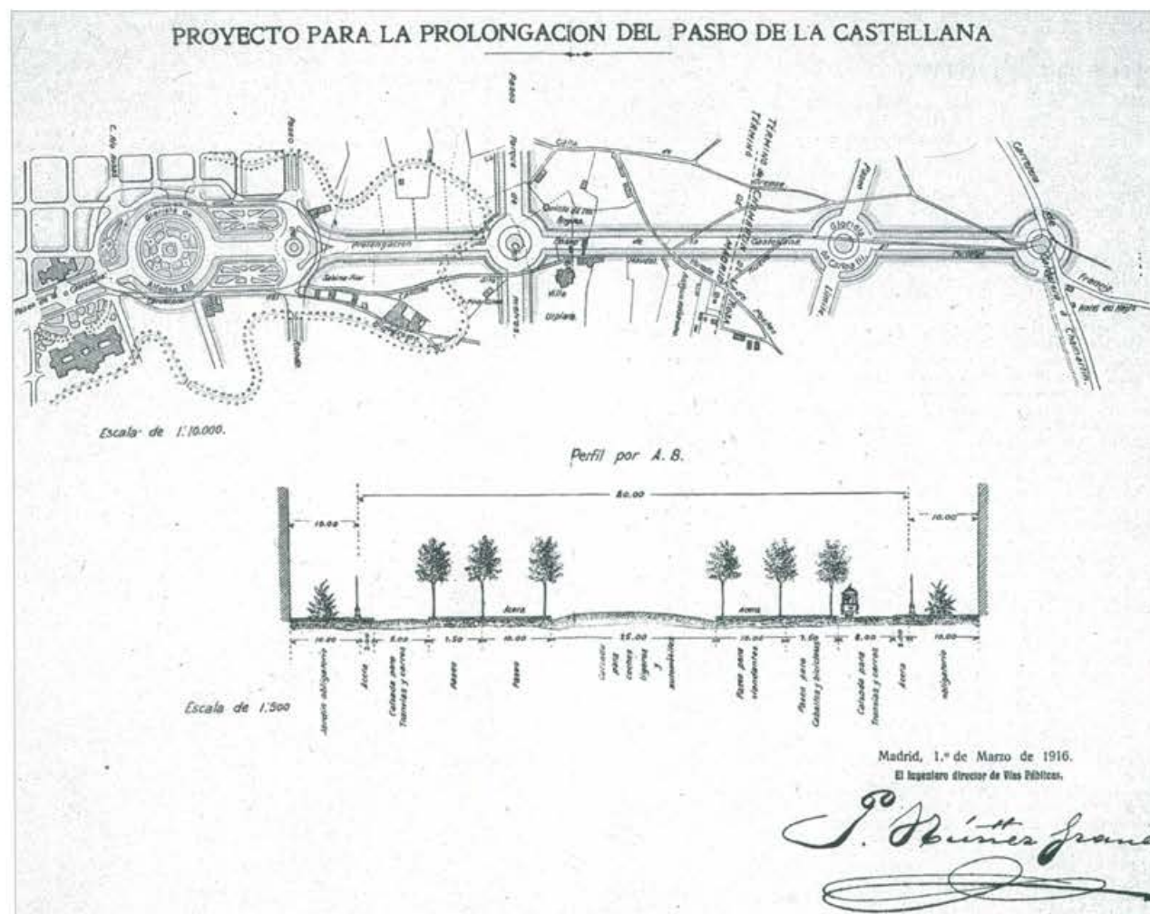
Proyecto para la prolongación del Paseo de la Castellana, P. Núñez Granés, 1916
