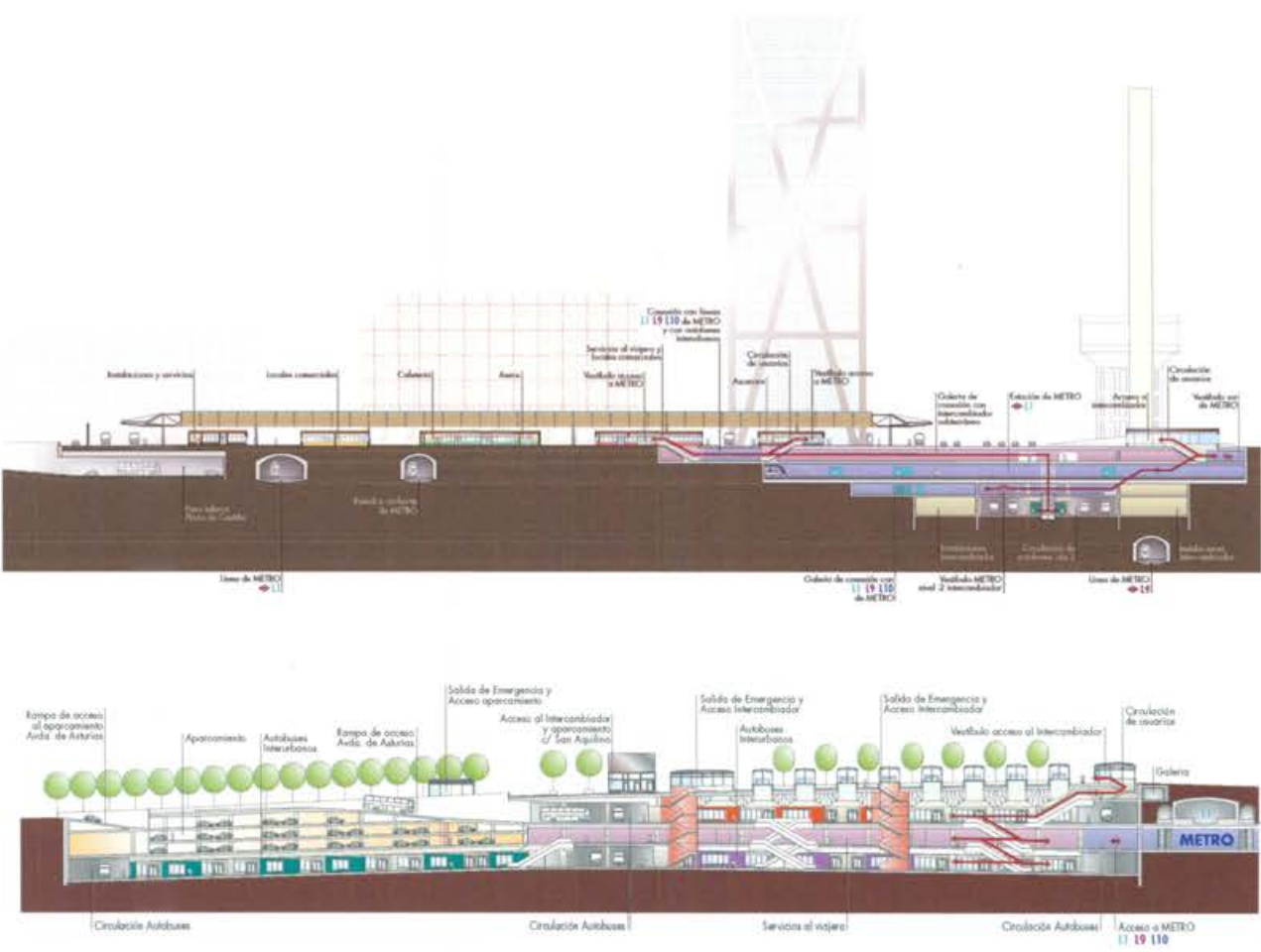
Intercambiador de plaza de Castilla [21:122]
