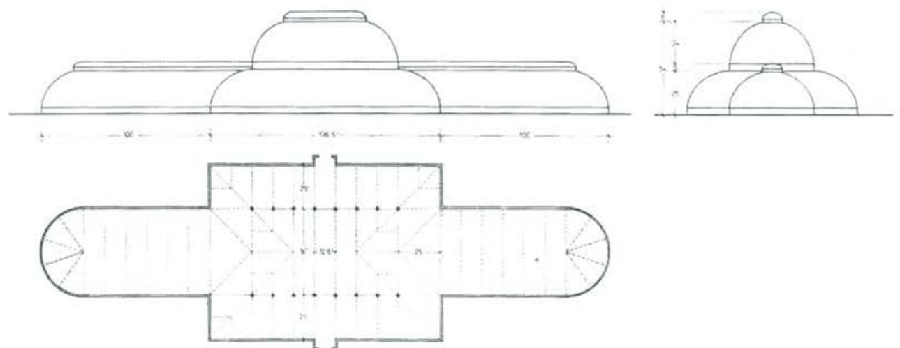
Planta y sección de PalmHouse, Kew Gardens (Richard Turner, 1844) 29
