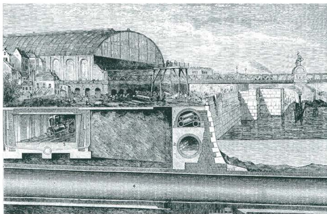
Victoria Embankment, sección, 1867 [61:159]
